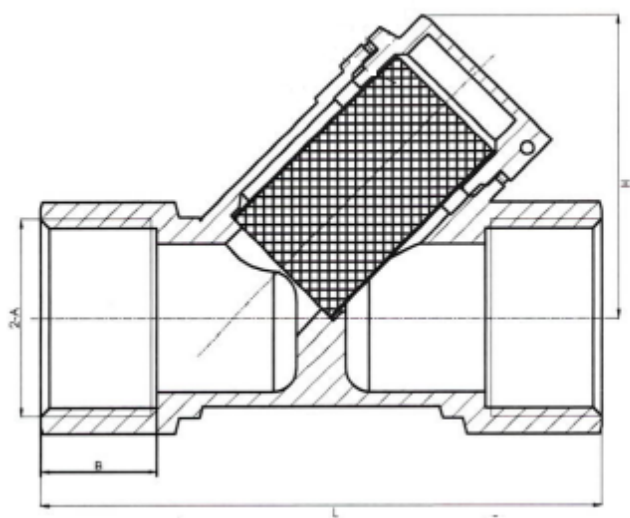
Габаритные размеры фильтров сетчатых FVR-R
