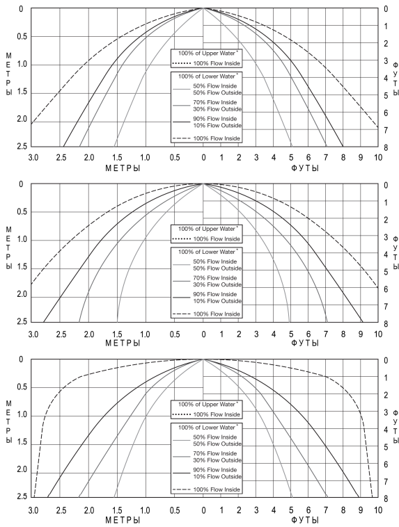
Рис. 4 Карта орошения оросителей модели TY7151 (K17-231) с вогнутой розеткой
