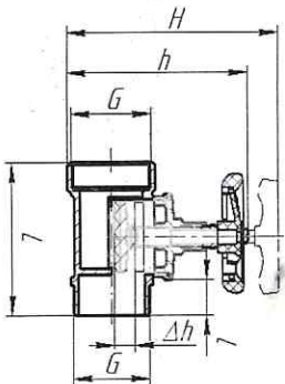
Рисунок 1- Внешний вид клапанов угловых моделей КПП, КТЧ, КПК и КППМ, КТЧМ, КПКМ
