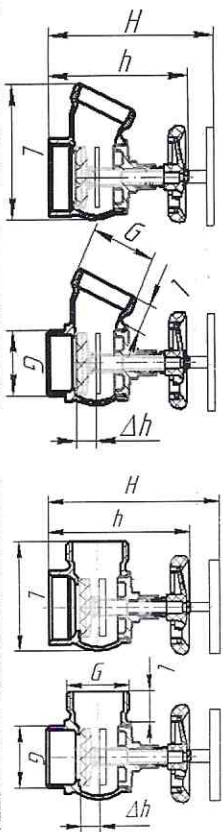
Рисунок 1- Внешний вид клапанов угловых моделей КПП, КТЧ, КПК и КППМ, КТЧМ, КПКМ
