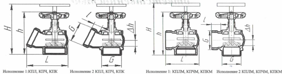
Рисунок 1—Внешний вид клапанов угловых моделей КПЛ, КПЧ, KPK и КПЛМ, КПЧМ, KPKM
